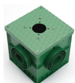
Socle en PVC 25 x 25 x 25 cm Ref 010904010184
